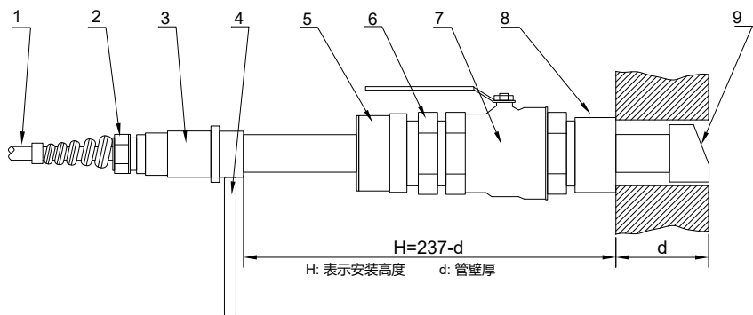
图 16 高温型插入式传感器结构图
